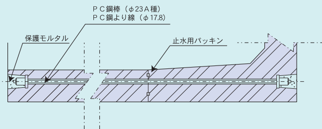
緊張及び接手部詳細図
