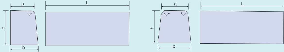
片面歩車道境界ブロック
